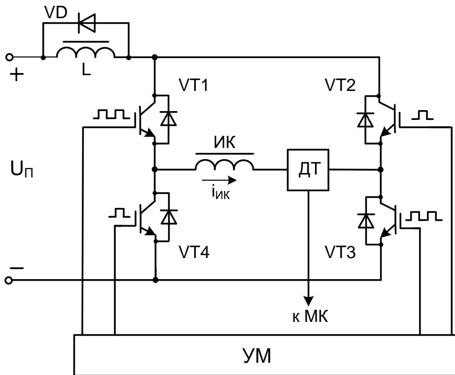
Рисунок 3. Электрическая схема мостового транзисторного преобразователя
