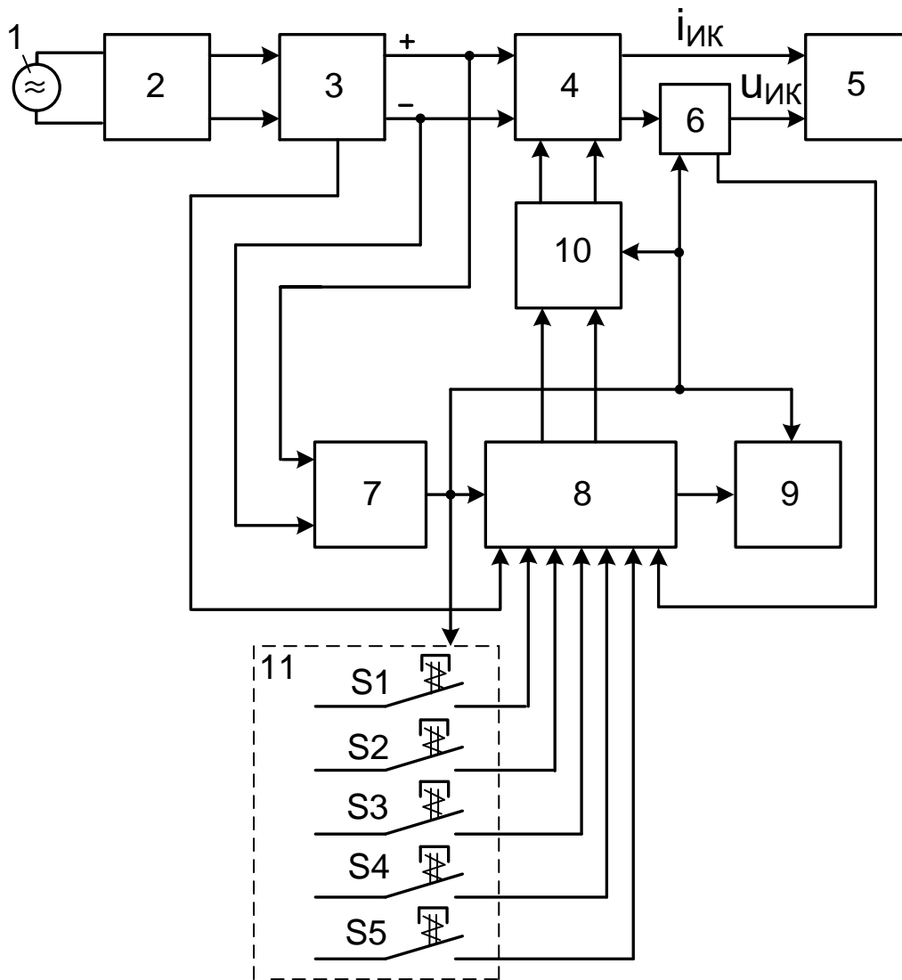
Рисунок 1. Упрощенная структурная схема устройства
