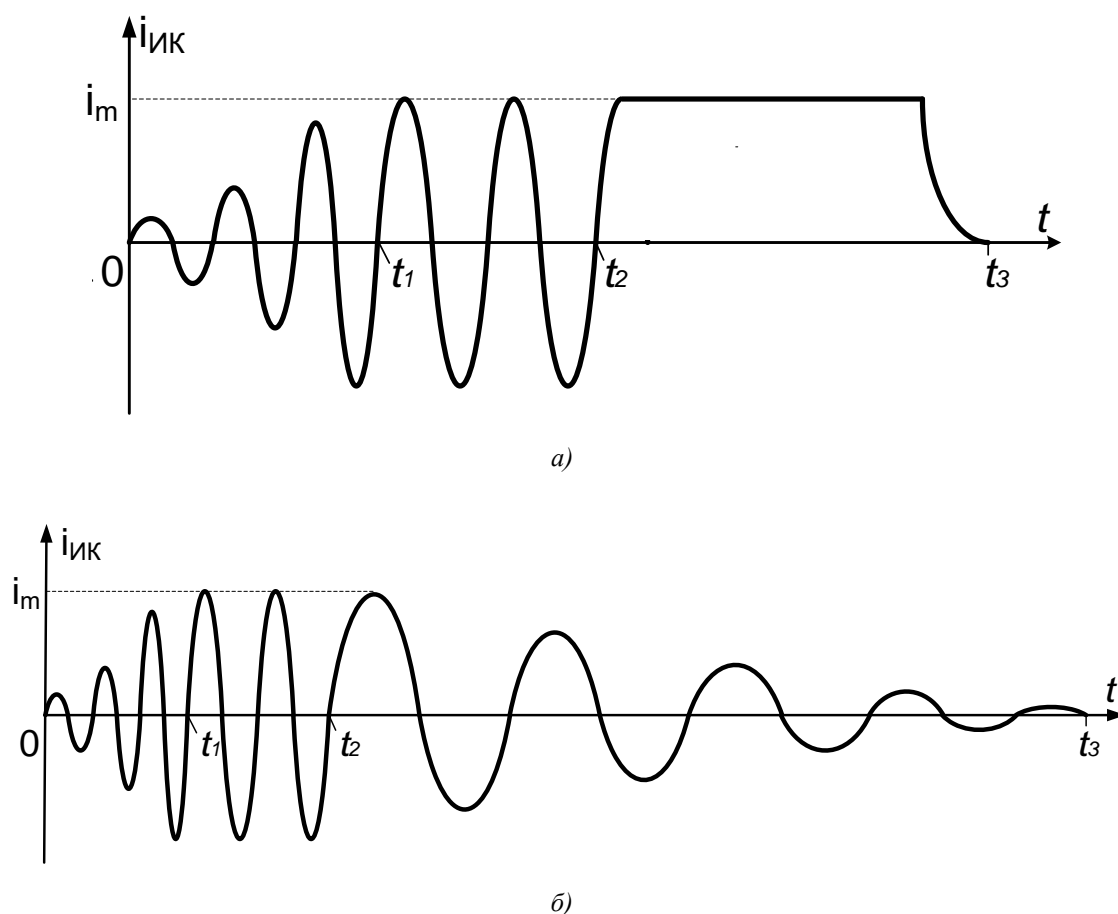
Рисунок 2. Временные диаграммы тока индуктивной катушки в процессе намагничивания (а) и размагничивания (б)
