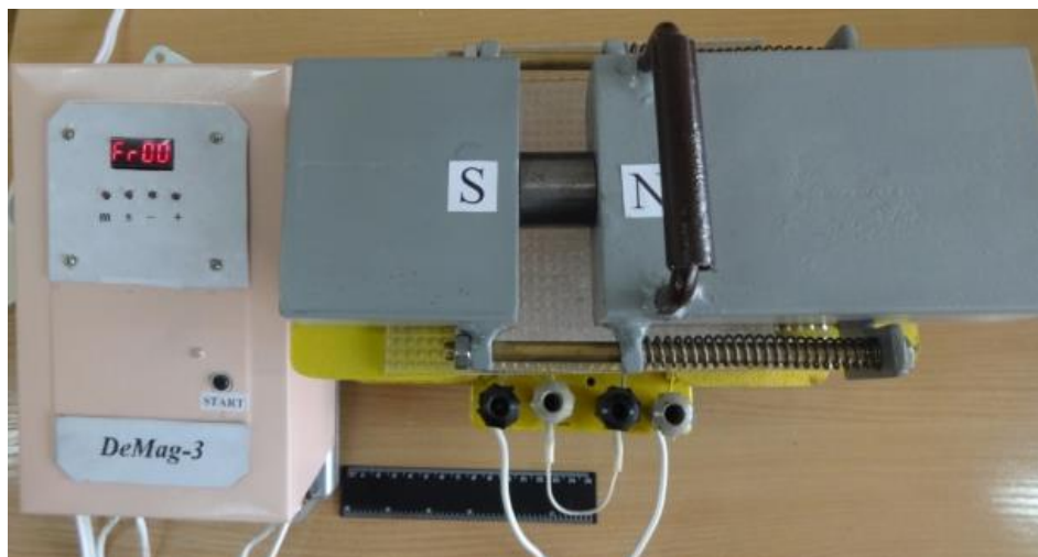
Рисунок 4. Фотоснимок устройства
